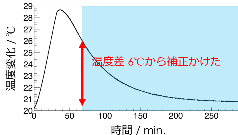
屈折率補正 あり
