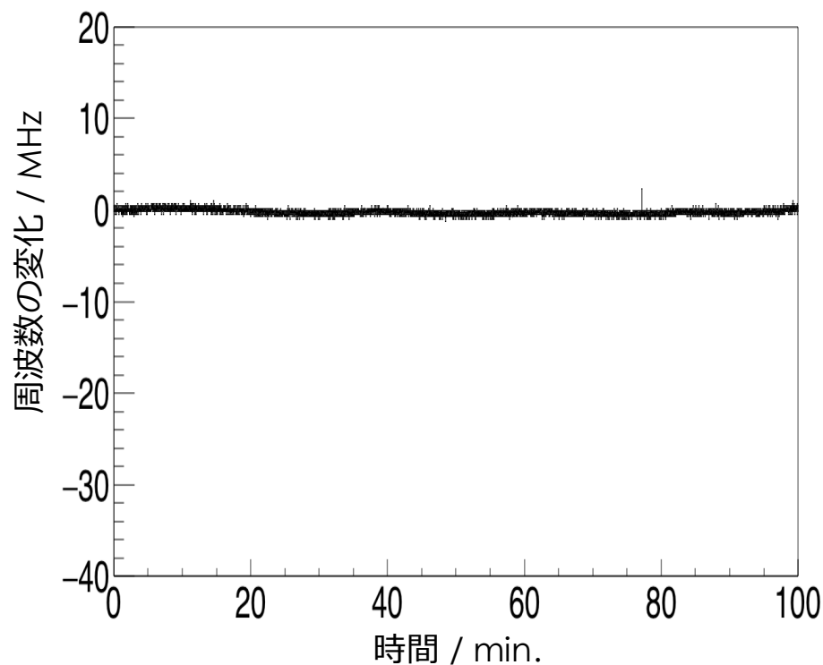
周波数安定化 (トランスファー共振器で安定性伝達)
