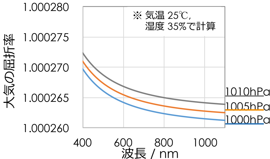
大気屈折率の波長・気圧依存性
